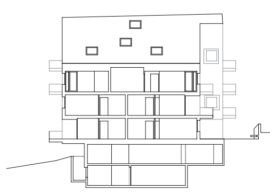
querschnitt
