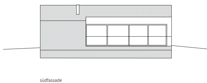
südfassade
