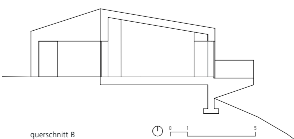
querschnitt B
